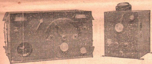
éléments du poste A.I.M. : Emetteur et boîte de commande.
