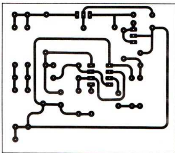
Figure 2. - Le circuit imprimé (échelle 1).
