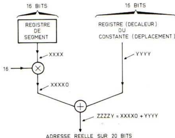
Fig. 3. - Procédure de calcul des adresses dans le 8088.
