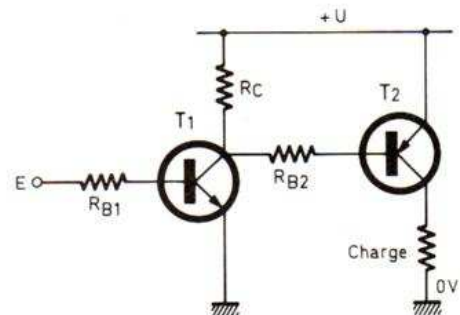
Fig. 10. - La charge a un point commun avec la masse.
