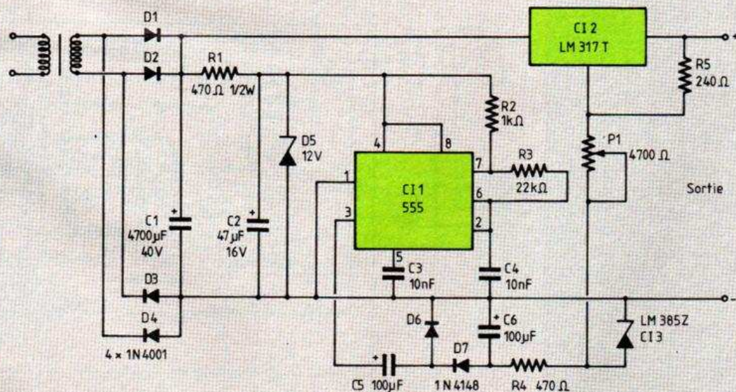
Figure 1. - Le schéma de principe de notre alimentation.
