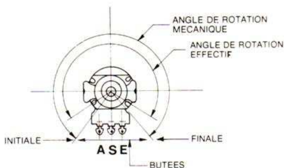
Figure 1a Angles de rotation pour les potentiomètres sans interrupteur ou avec un interrupteur « push-push ».
