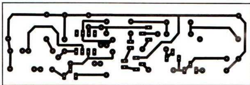
Figure 2. - Le circuit imprimé (échelle 1).
