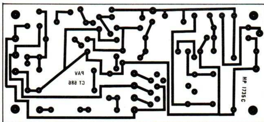
Figure 3. – Circuit imprimé, vu côté cuivre, échelle 1.
