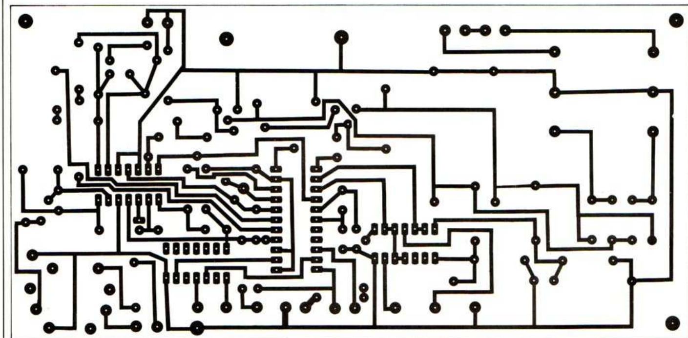
Fig. 2. - Circuit imprimé, vu côté cuivre, échelle 1.
