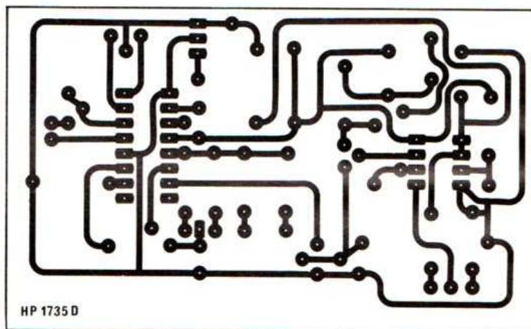
Figure 2. - Le circuit imprimé à l'échelle 1.
