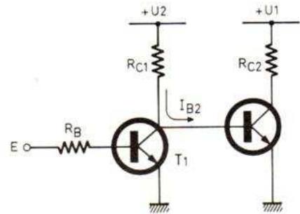
Fig. 9. - Commutation à deux étages.
