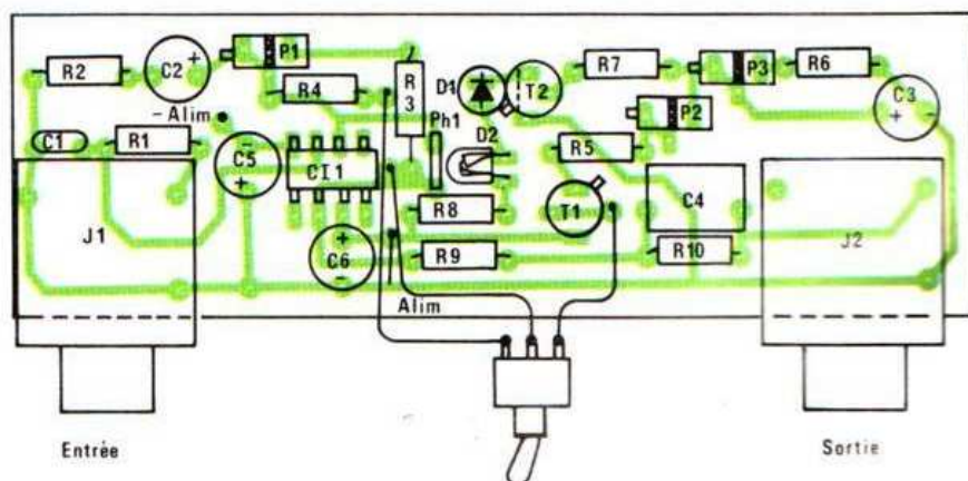
Figure 3. - Disposition des composants sur le circuit imprimé.
