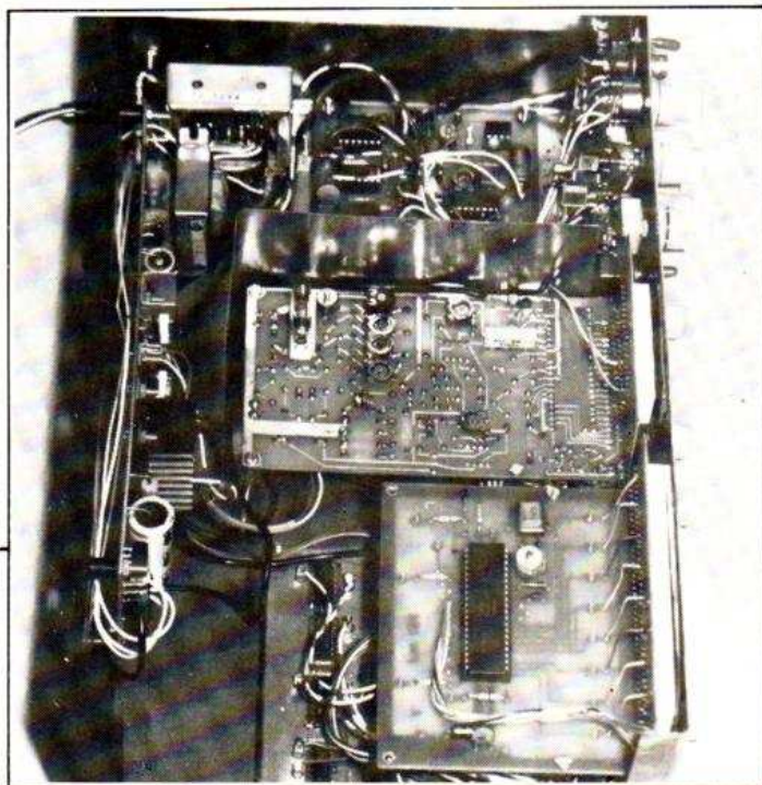
Photo 14 Le circuit est disposé dans le coffret. Notez la disposition de la tôle de blindage.
