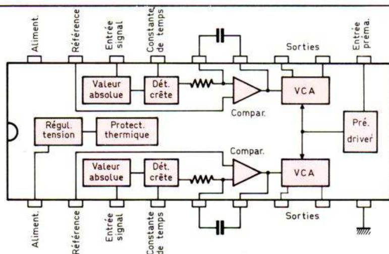
Figure 5. — Synoptique du circuit intégré \mu PC 1297 CA Dolby HX Pro.
