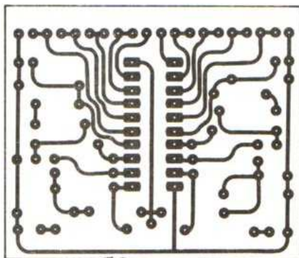
Figure 12. - Le circuit imprimé.
